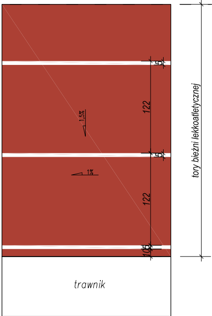
szczegóły nawierzchni bieżni lekkoatletycznej skala 1:50
